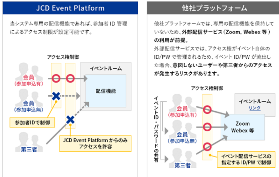
「JCD Event Platform」配信機能のアクセス制御
